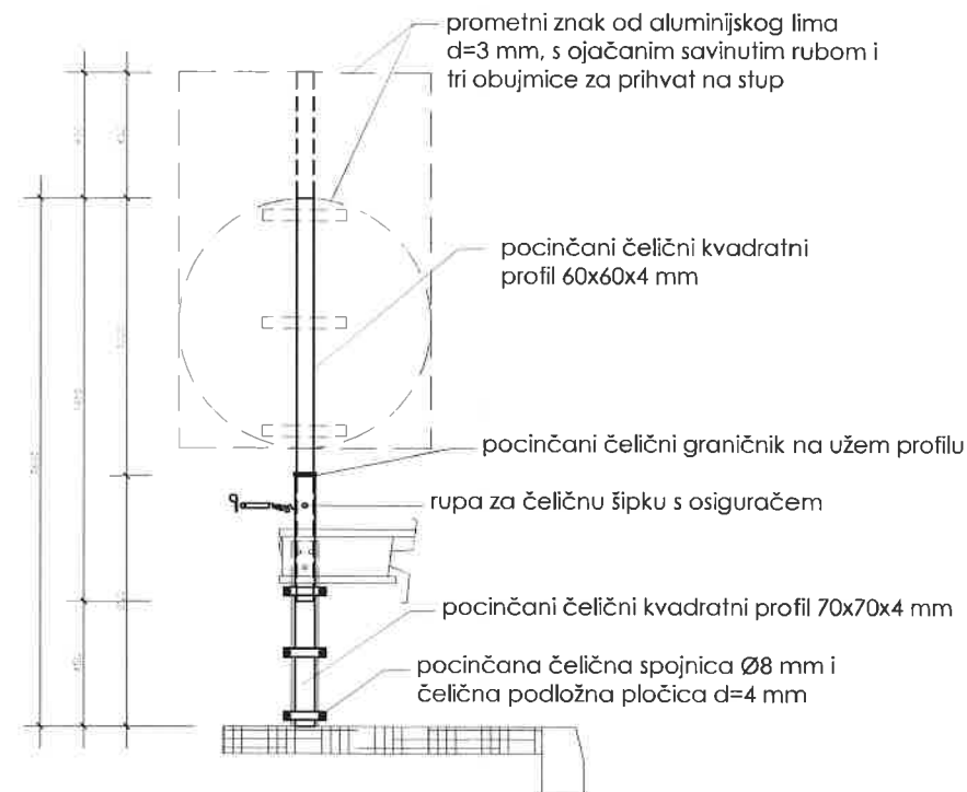
MONTAŽA NA ODBOJNU OGRADU
