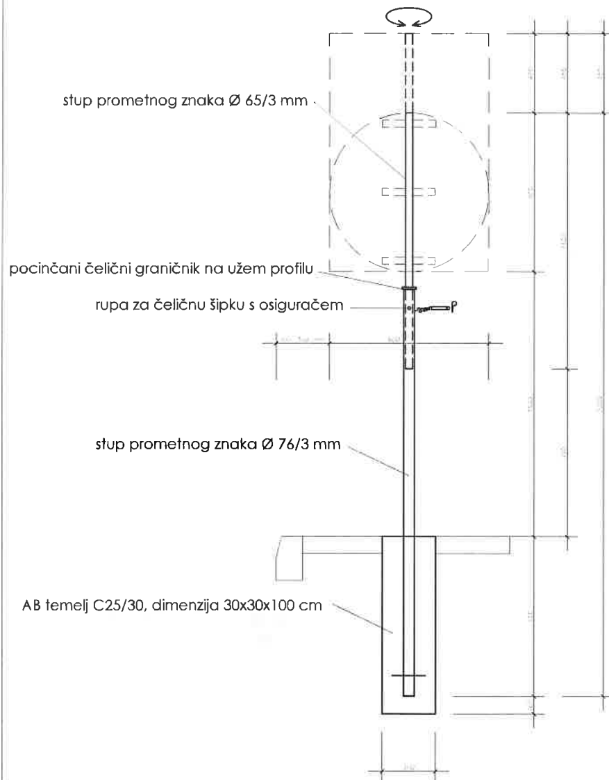
KLASIČNA MONTAŽA - zakretna ploča znaka -
