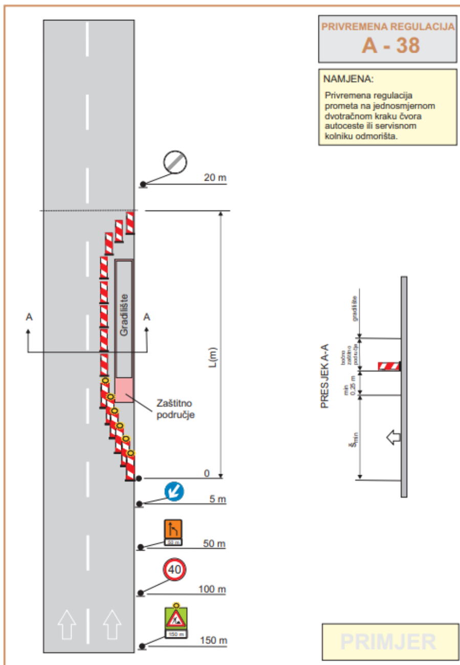
Slika 3 Privremena regulacija prometa tip A-38 (Pravilnik o privremenoj regulaciji prometa i označavanju te osiguranju radova na cestama (NN 92/19))
