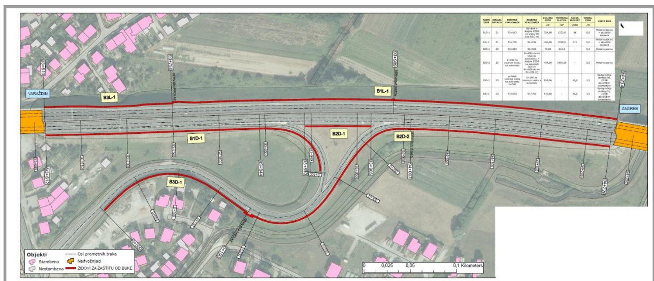
Slika 1. Pregledna situacija zidova za zaštitu od buke od 93+600 do 94+250
