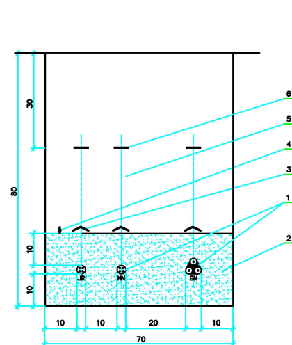
PRESJEK KABELSKOG ROVA ZA POLAGANJE KABELA NAZIVNIH NAPONA U0/U=0,6/1 kV I U/U=12/20 kV U ZAJEDNIČKI ROV
