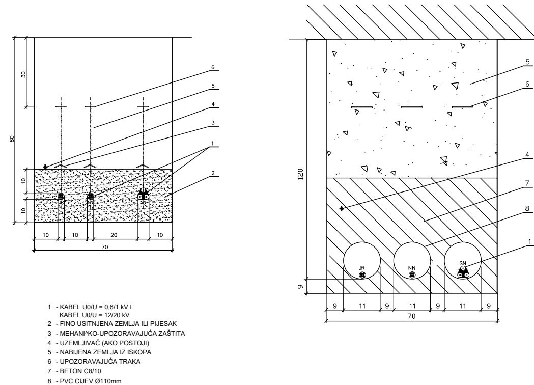
PRESJEK KABELSKOG ROVA ZA POLAGANJE KABELA NAZIVNIH NAPONA U0/U=0,6/1 kV I U/U=12/20 kV U ZAJEDNIČKI ROV
