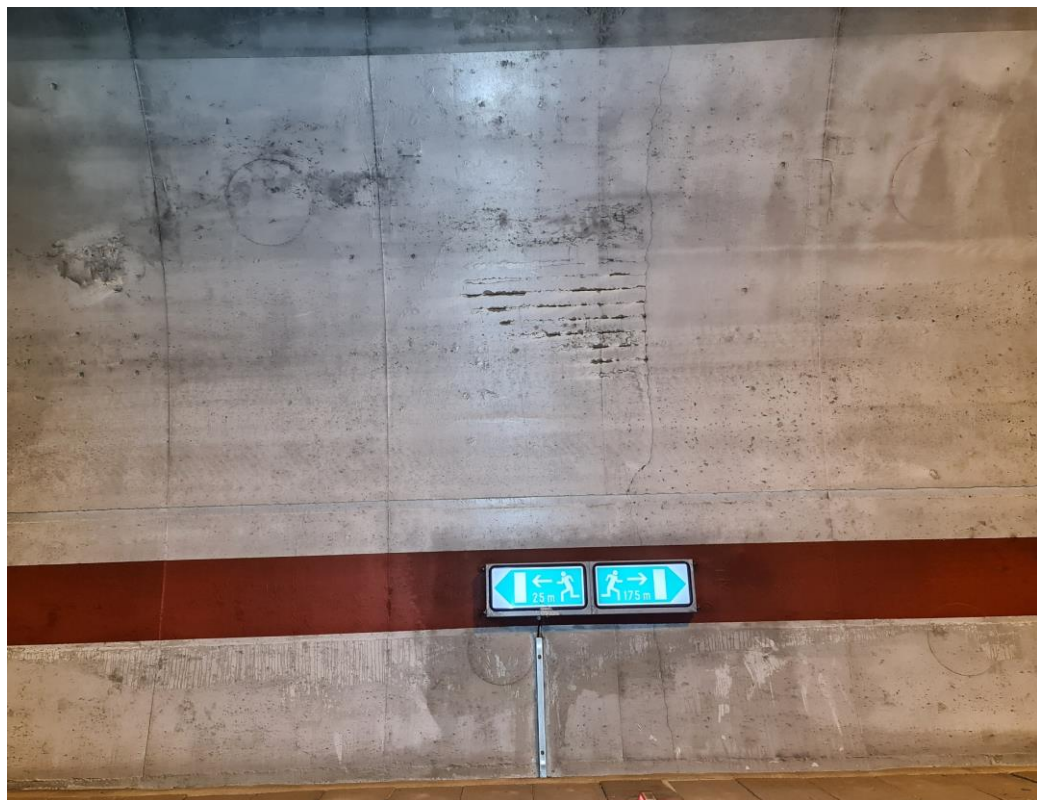
Slika 29: Kampada 35 - RADIJALNA PUKOTINA, KOROZIJA ARMATURE
