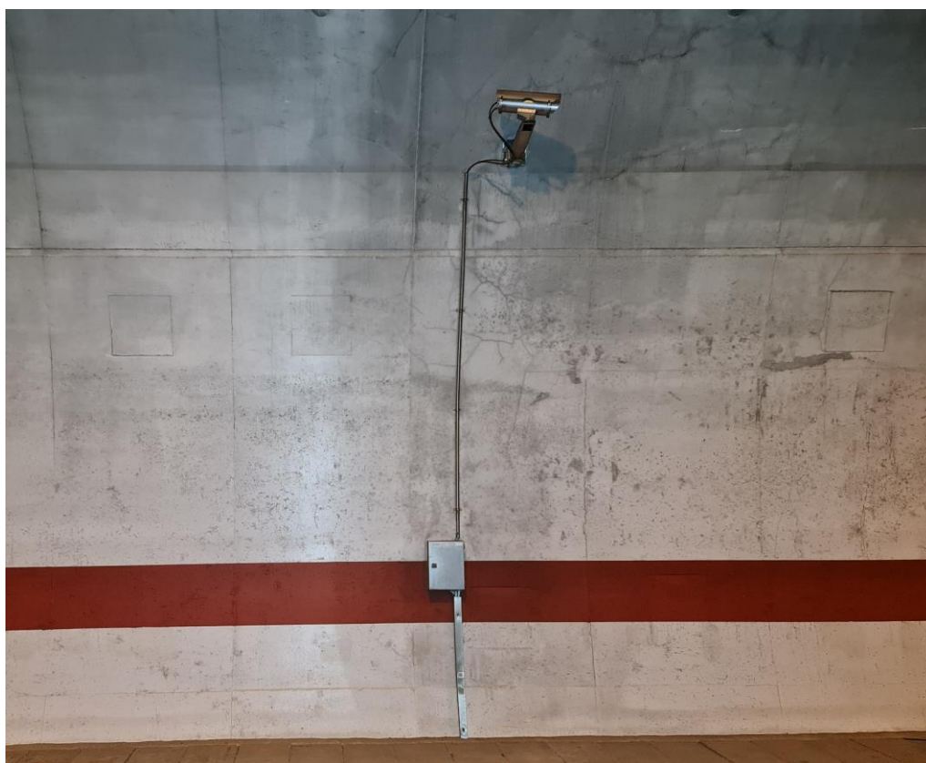
Slika 15: Kampada 138 - MREŽASTE PUKOTINE
