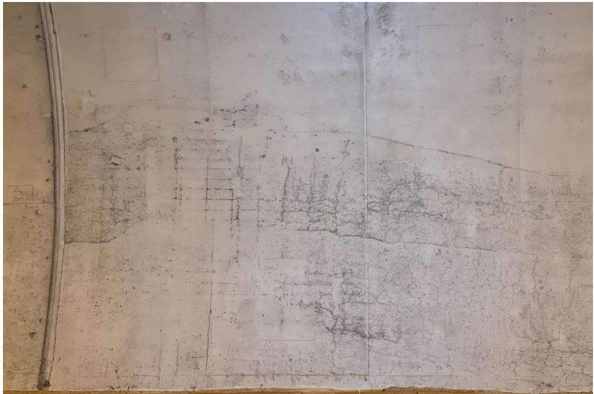
Slika 7: Kampada 36 - NEDOSTATAK ZAŠTITNOG SLOJA
