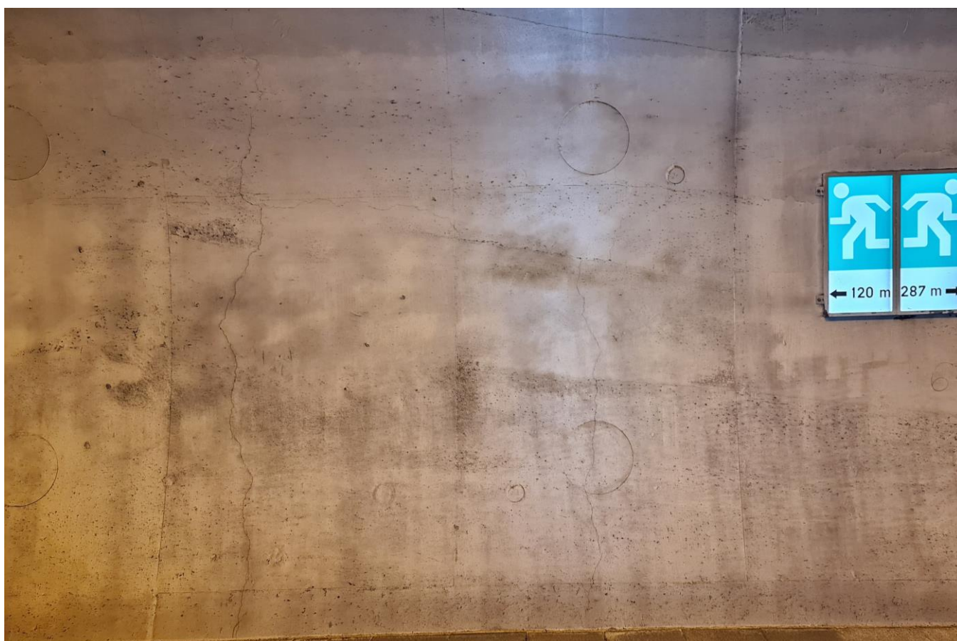
Slika 6: Kampada 63 - RADIJALNE PUKOTINE
