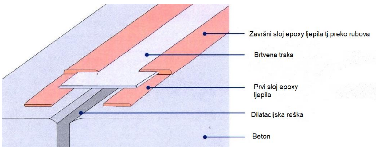
Slika 7: Skica načina ugradnje brtvene trake na reški betonske obloge između dvije kampade
