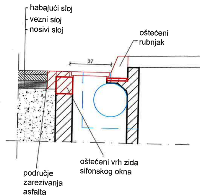
PRESJEK C-C
