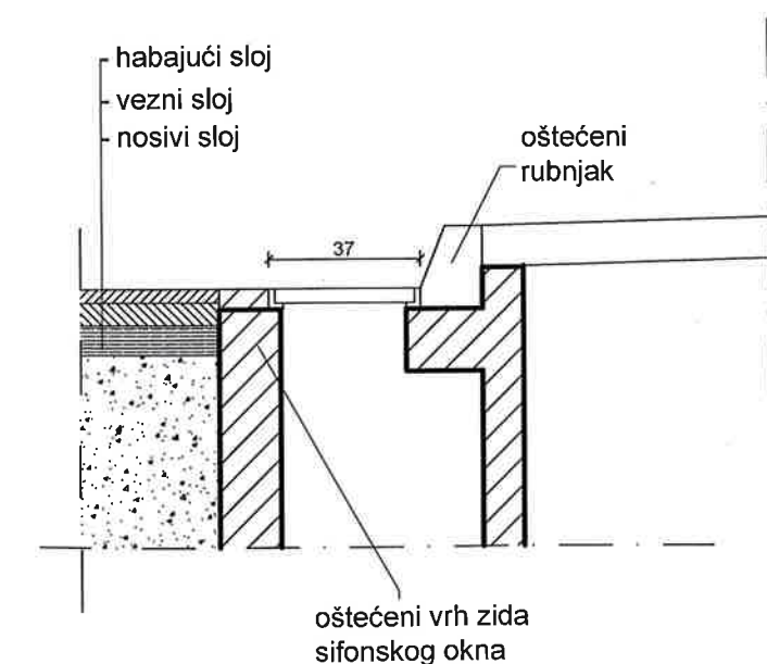
PRESJEK C-C
