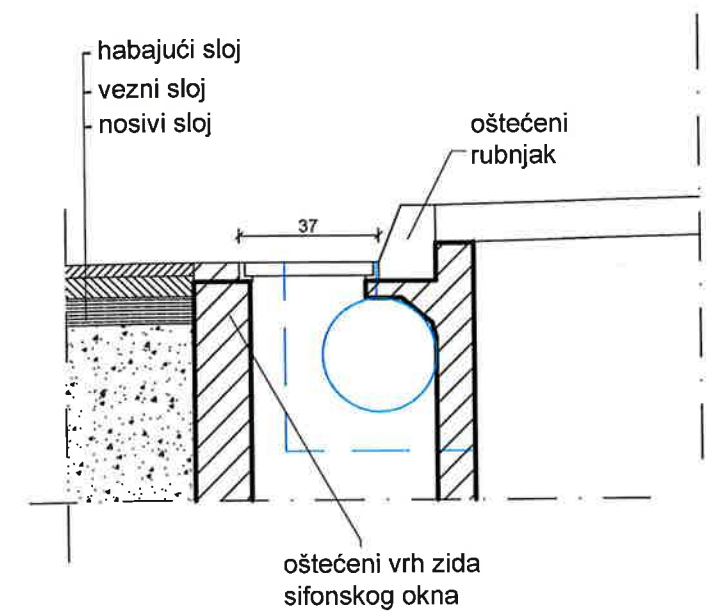
PRESJEK B-B
