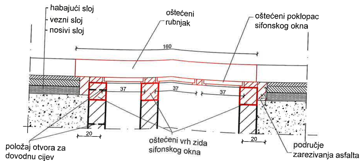
PRESJEK A-A
