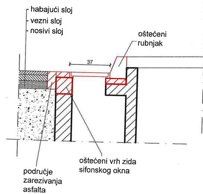
PRESJEK C-C
