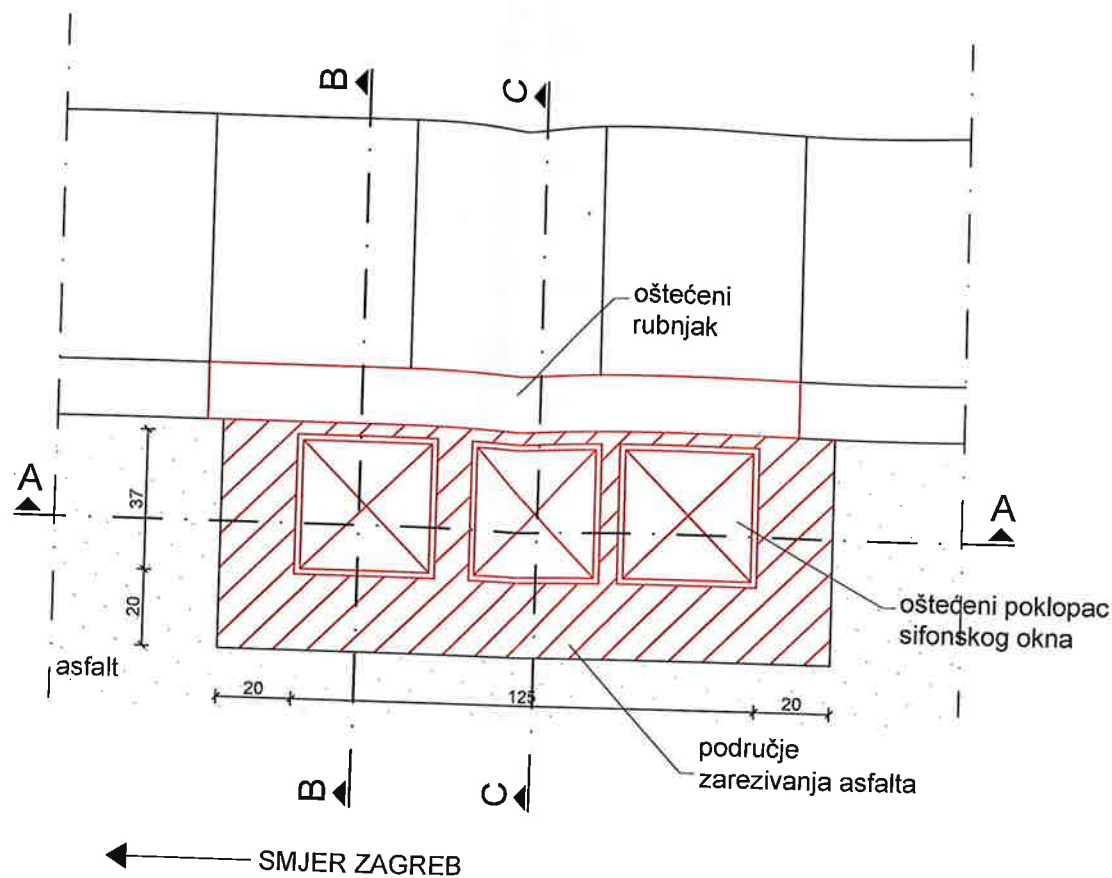
TLOCRT
