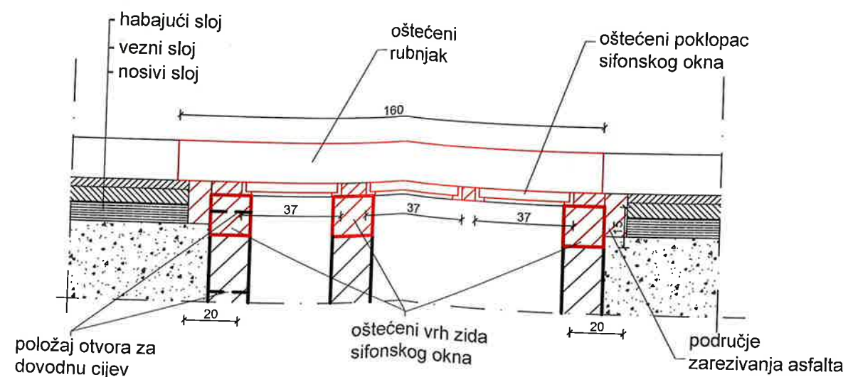
PRESJEK A-A
