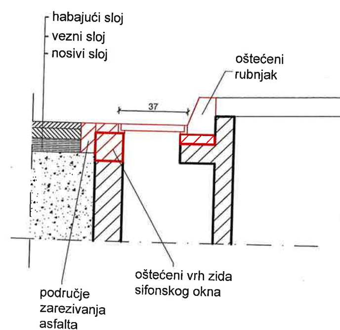
PRESJEK C-C
