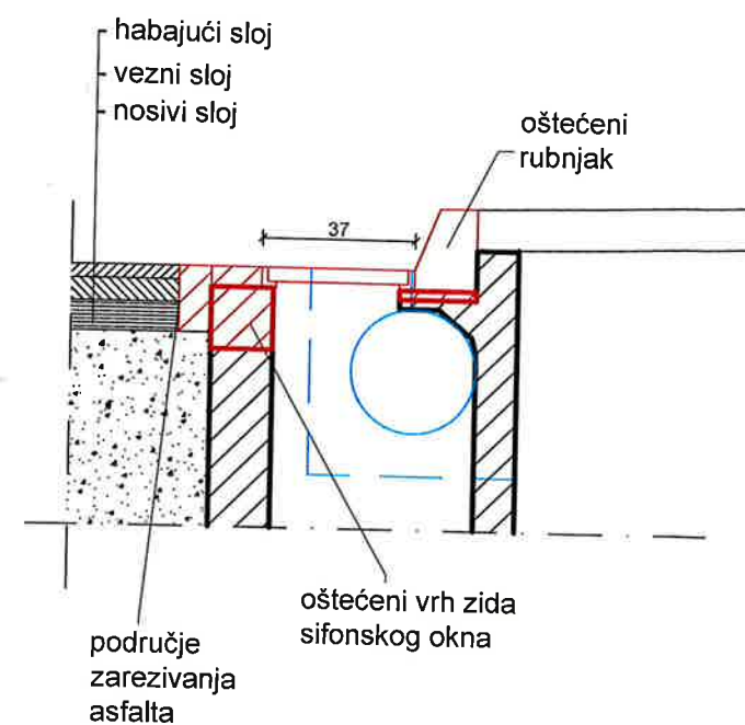
PRESJEK C-C
