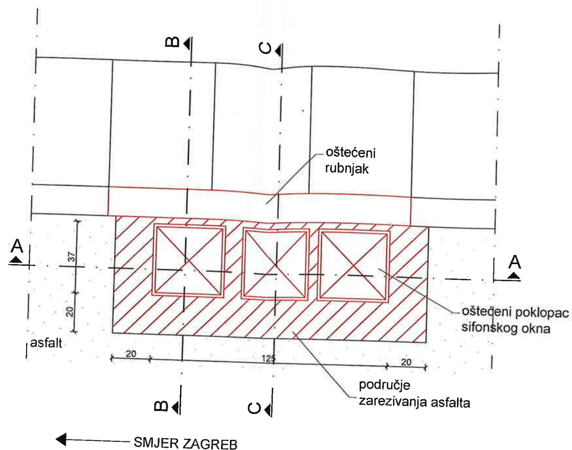
TLOCRT
