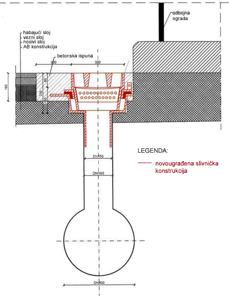
PRESJEK A-A
