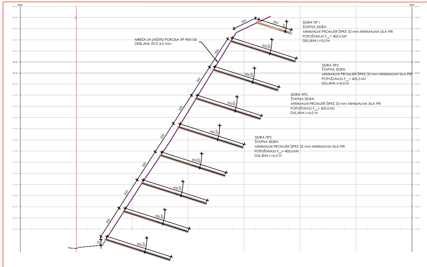
PRESJEK 34 (STAC. 0+330.00)
