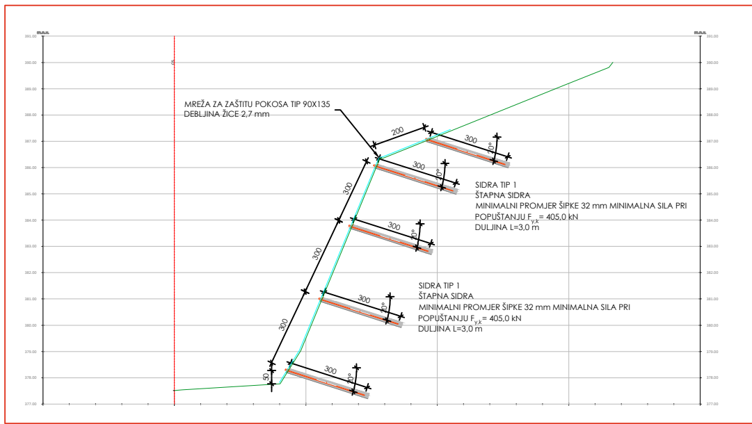
PRESJEK 21 (STAC. 0+200.00)
