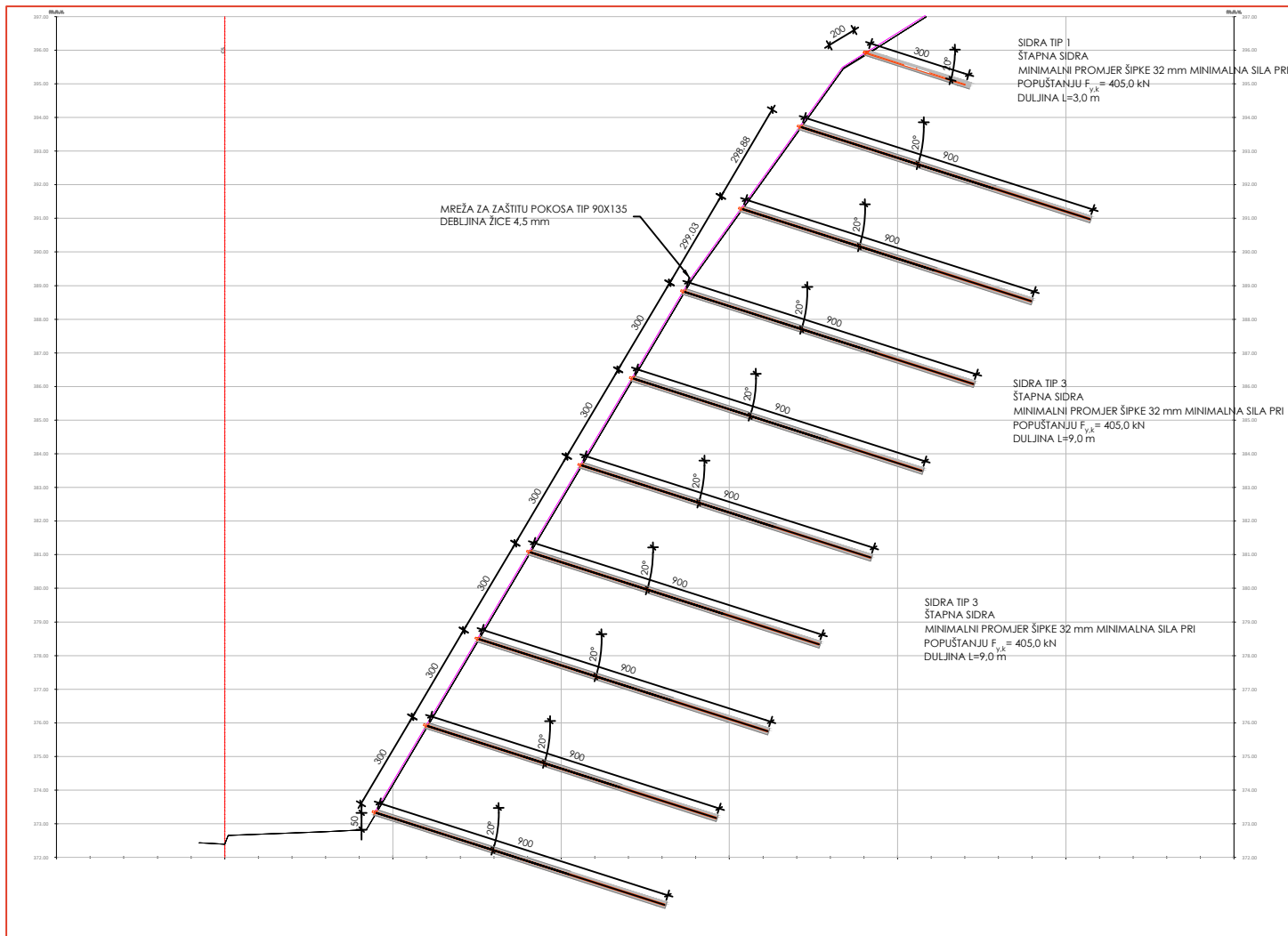
PRESJEK 21 (STAC. 0+200.00)
