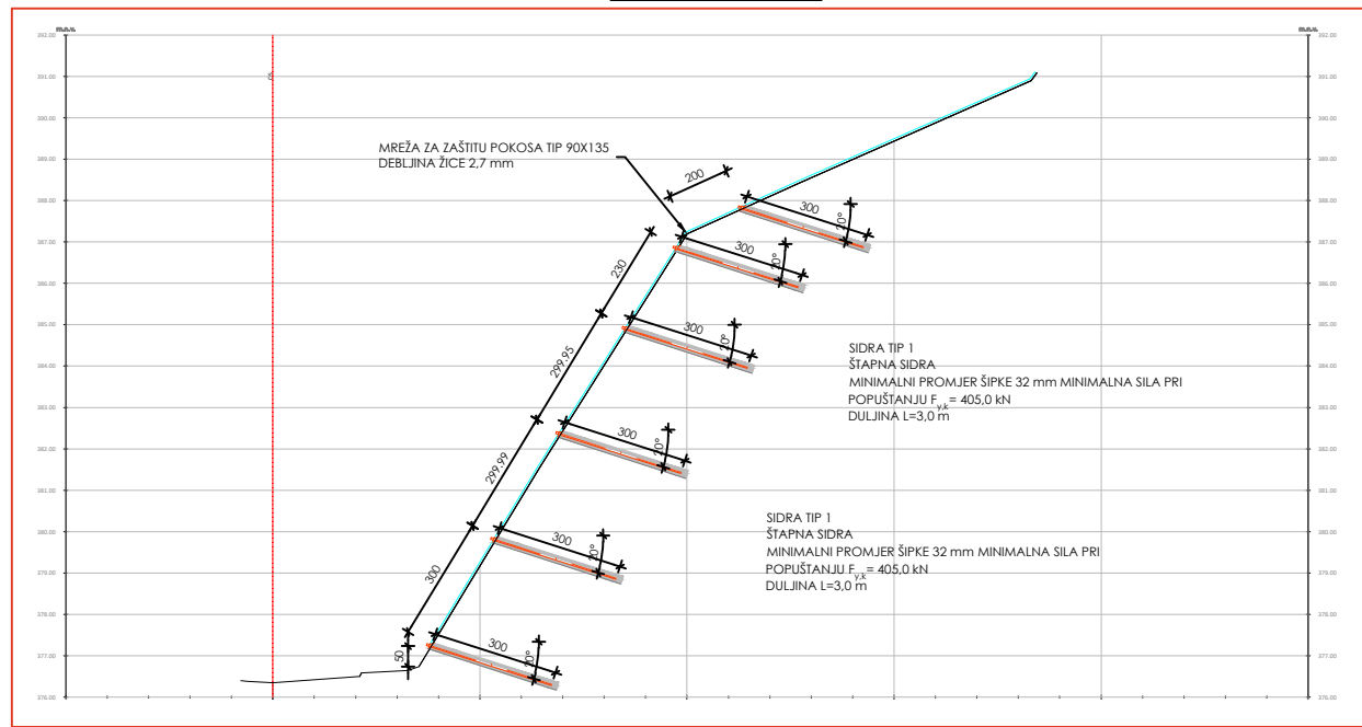
PRESJEK 11 (STAC. 0+100.00)
