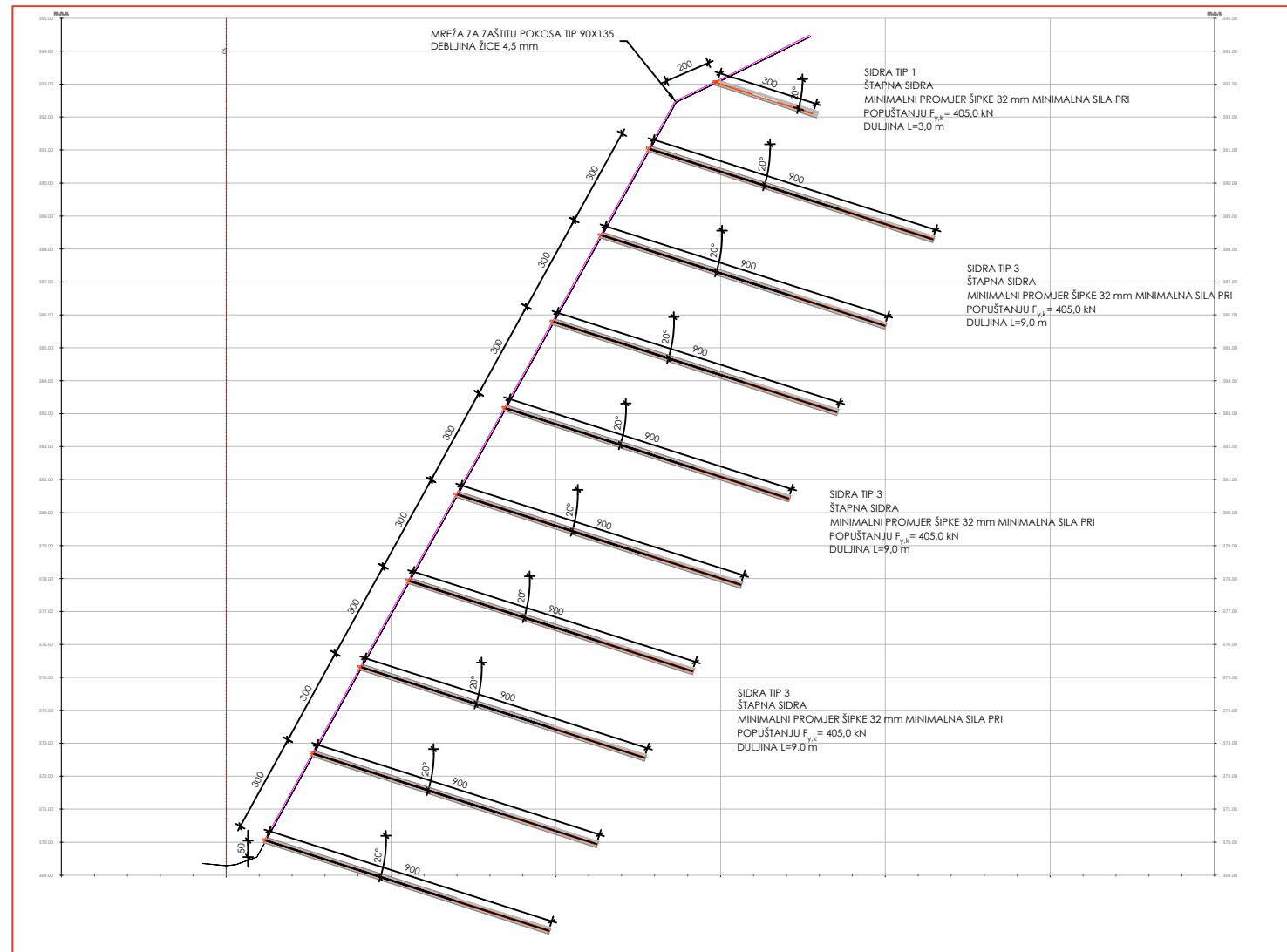
PRESJEK 29 (STAC. 0+280.00)
