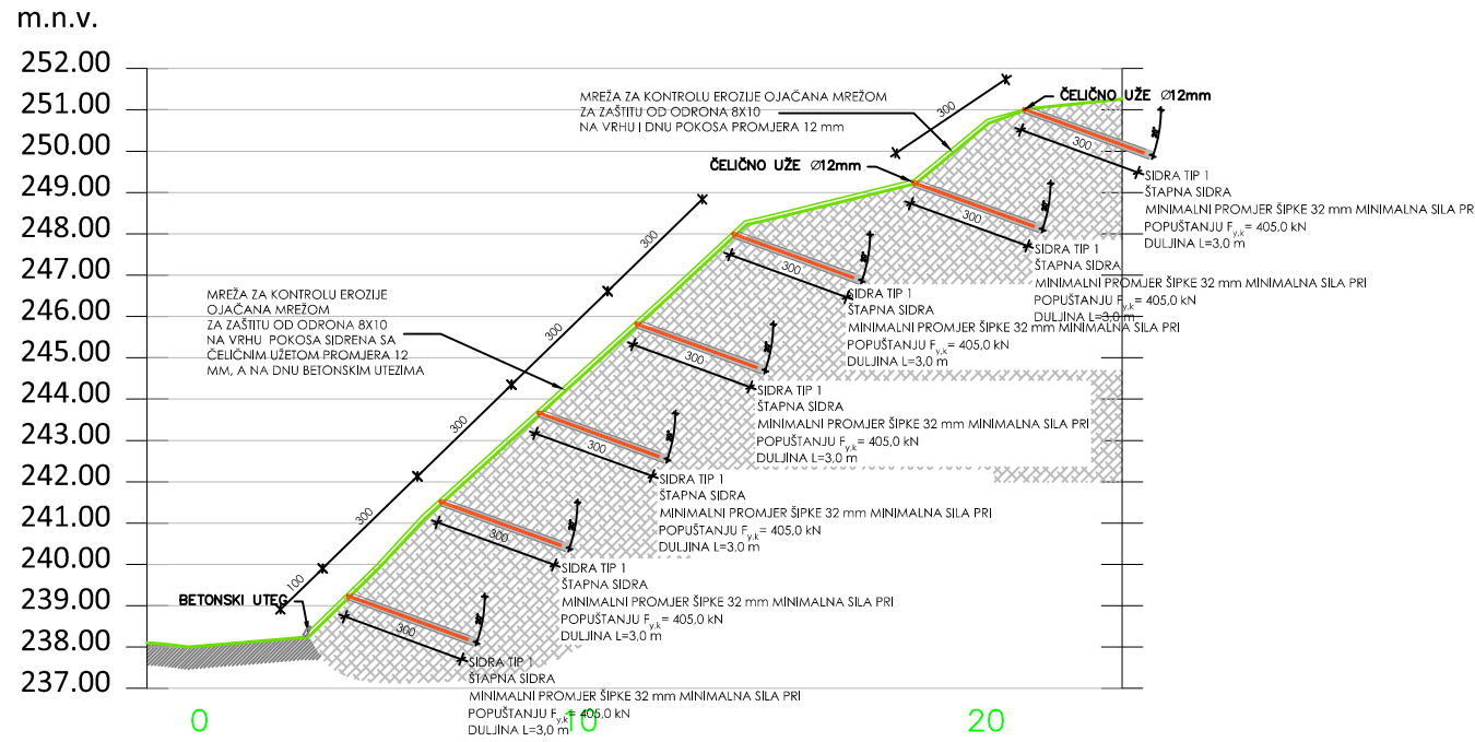
PRESJEK 1 (STAC. 0+698.00)
