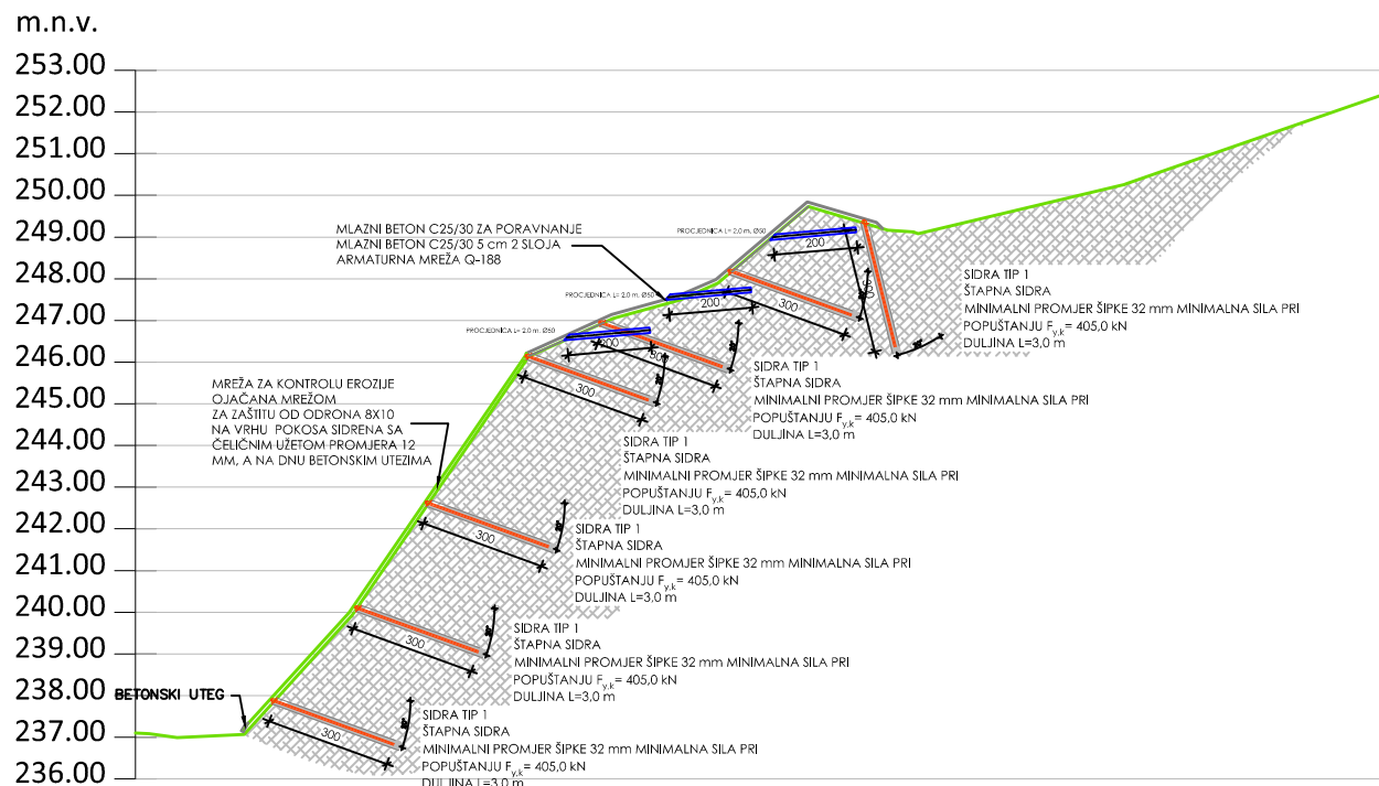
PRESJEK 5 (STAC. 0+438.00)
