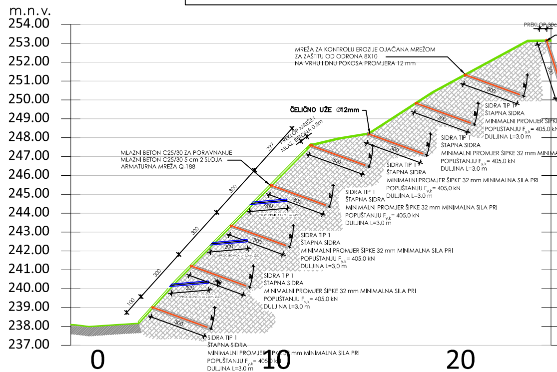
PRESJEK 2 (STAC. 0+678.00)
