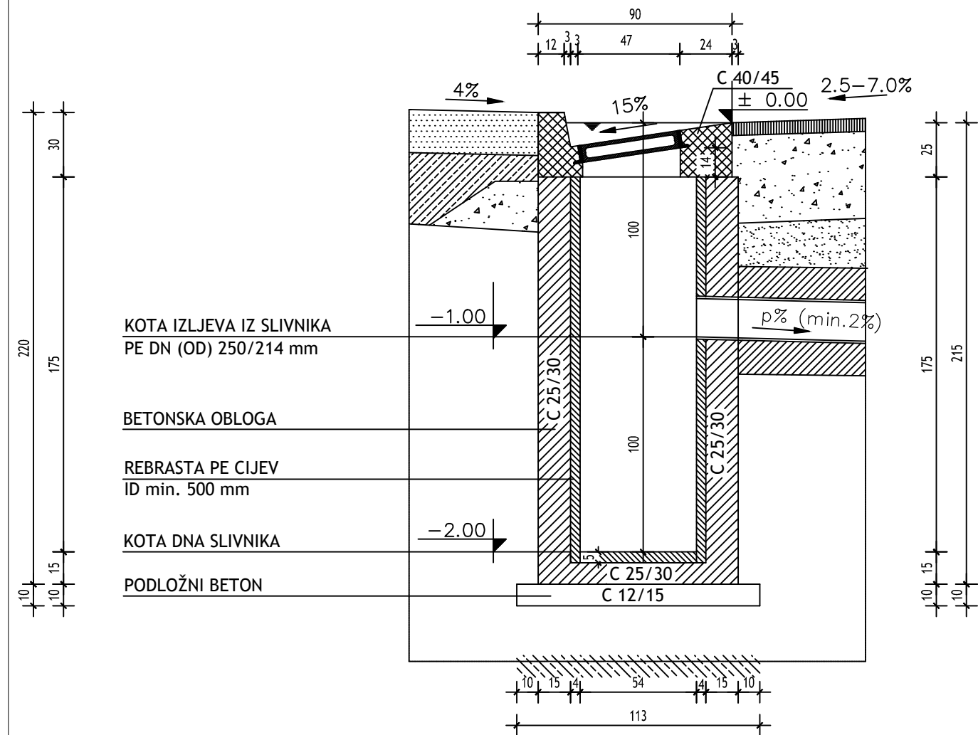
PRESJEK A-A
