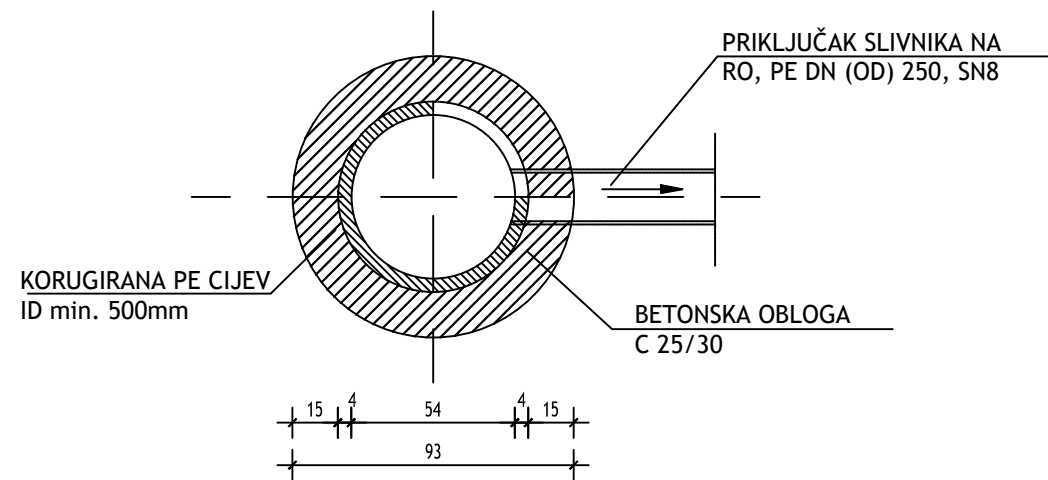
PRESJEK C-C
