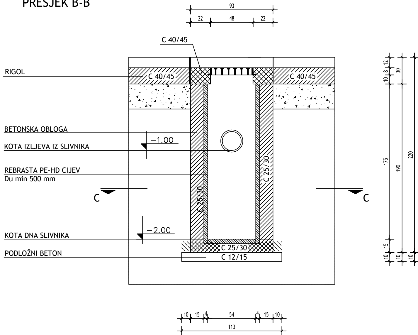
PRESJEK B-B
