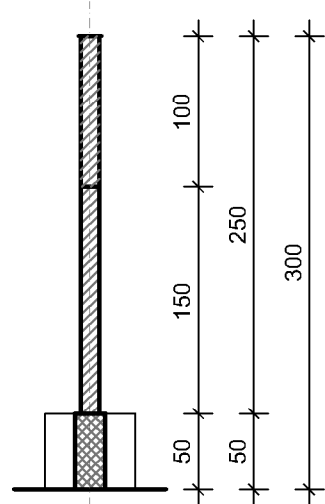
PRESJEK 5 - 5
