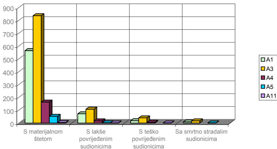
Broj nesreća u 2009. po autocestama
